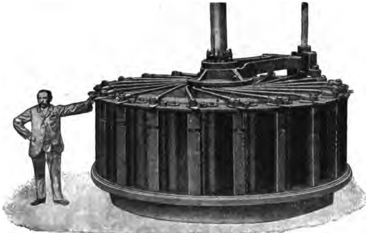
Fig. 30. Leitapparat der Francis-Turbine von Bregleb, Hansen & Co., Gotha.
